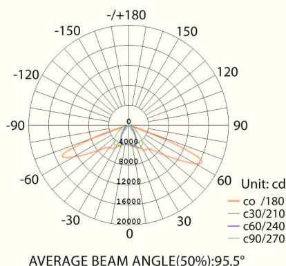
Кривая силы света:
