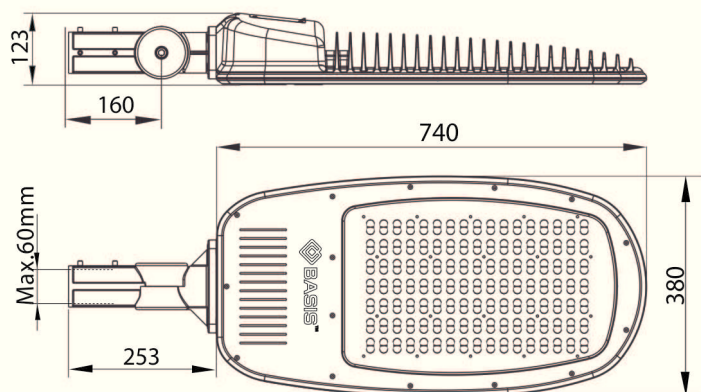
Размеры:
