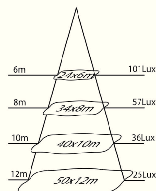
График освещенности:
