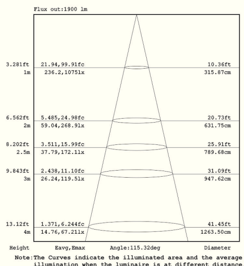
График освещенности:
